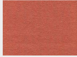
Turn CSE26
